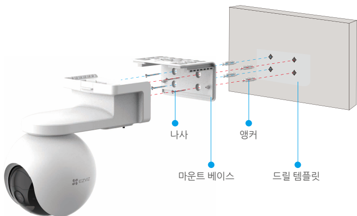
그림 2 벽 장착
