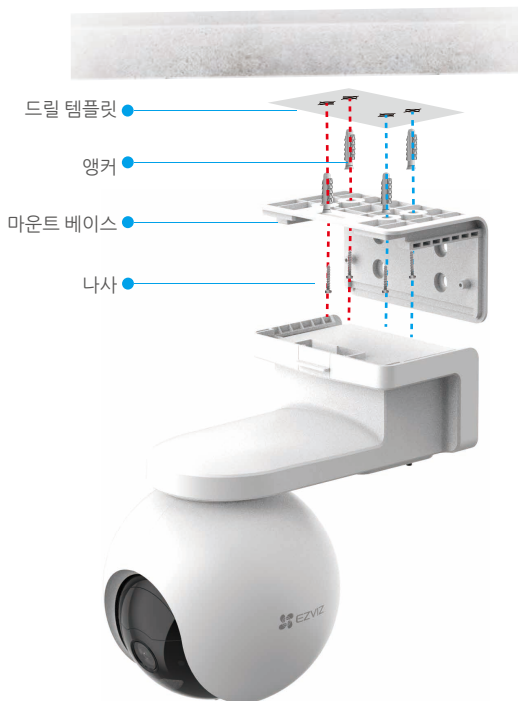
그림 1 천장 장착
